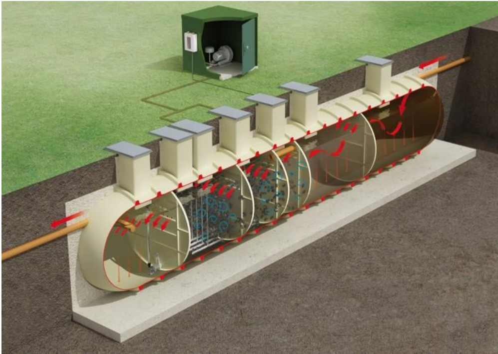
Na zdjęciu: Innowacyjne systemy oczyszczania ścieków EnviroSafe
