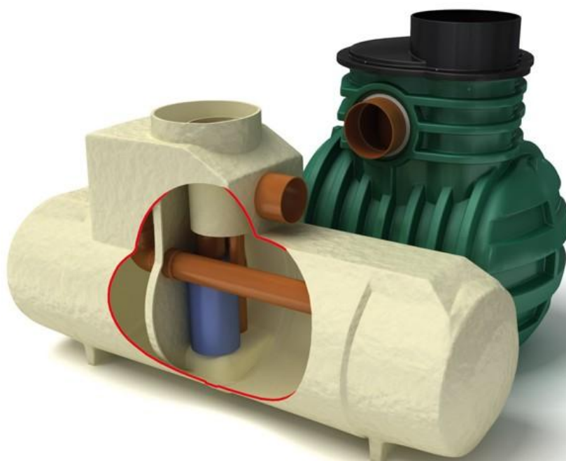
Na zdjęciu: Separatory substancji ropopochodnych
