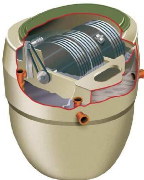
Na zdjęciu: Biologiczna, przydomowa oczyszczalnia BioDisc
